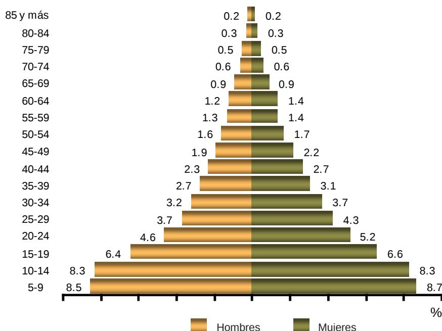
Estructura por edad y sexo de la población que habla tlapaneco, 2005
